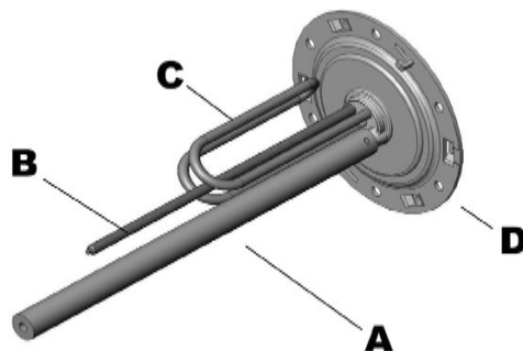
Afbeelding 1 – Dompelweerstand + magnesiumanode
